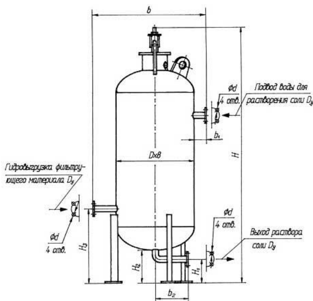
Рис.1. Конструкция солерастворителей Ду 500, 700, 1000 типа С.
